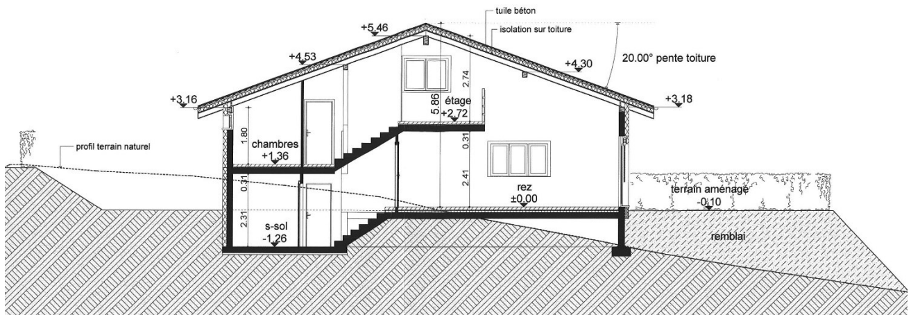
COUPE NORD-SUD
