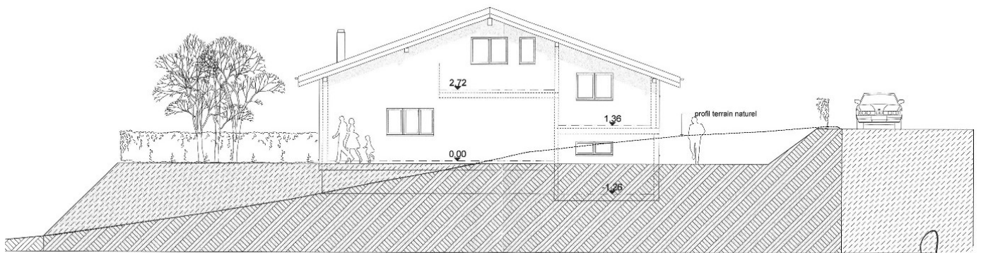
FACADE OUEST
