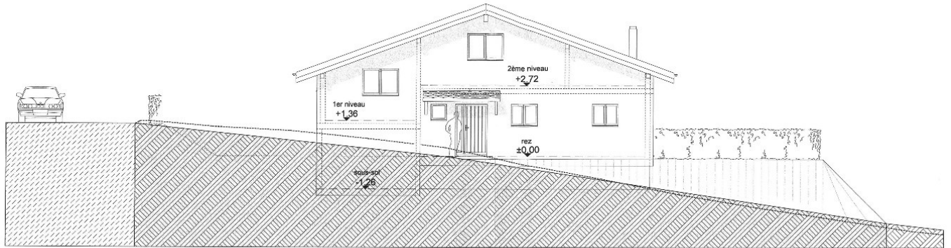
FACADE EST
